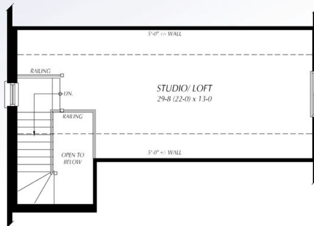
OPTIONAL LOFT FLOOR PLAN
