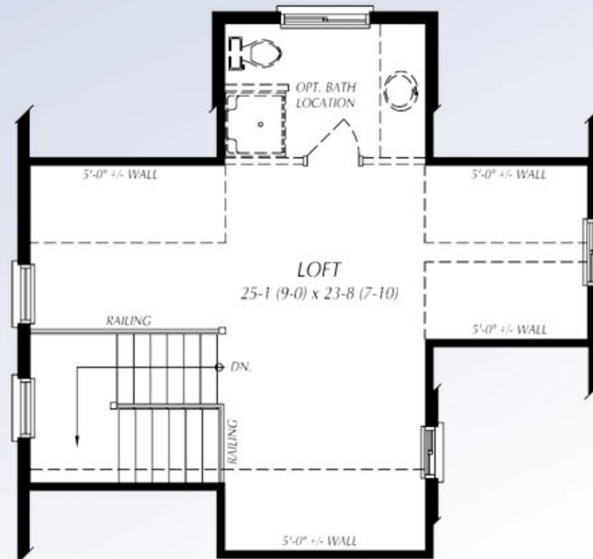
OPTIONAL LOFT FLOOR PLAN
