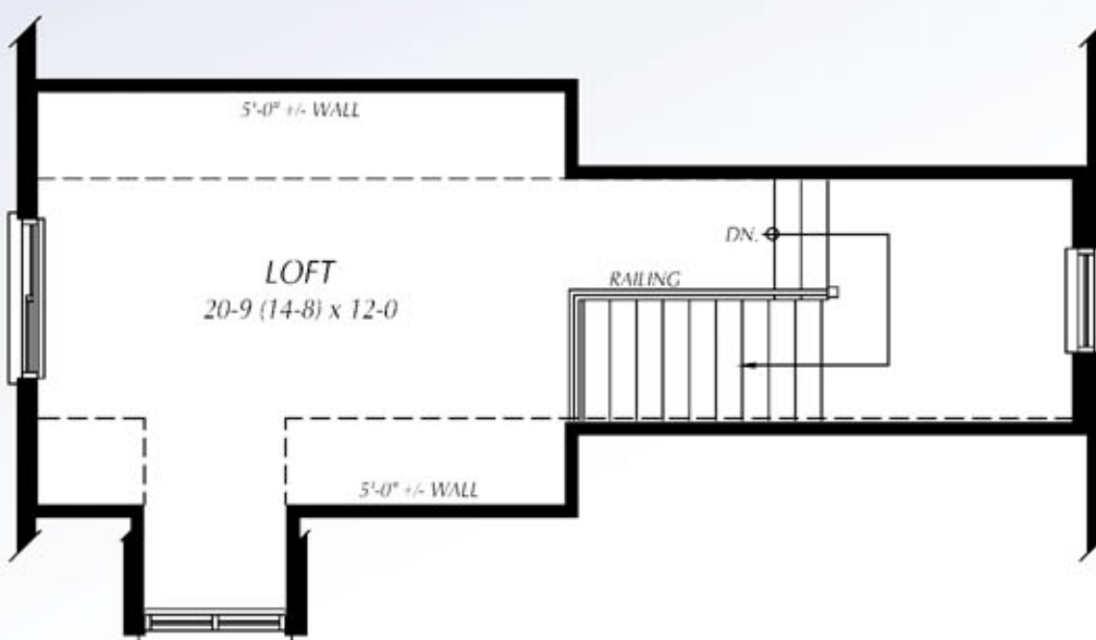
OPTIONAL LOFT FLOOR PLAN
